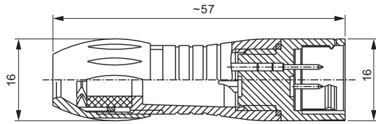
插槽式电缆接头, 电缆直径 4-6mm 针数 3, 5, 8
