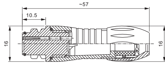
针式电缆接头, 电缆直径 4-6mm 针数 3, 5, 8
